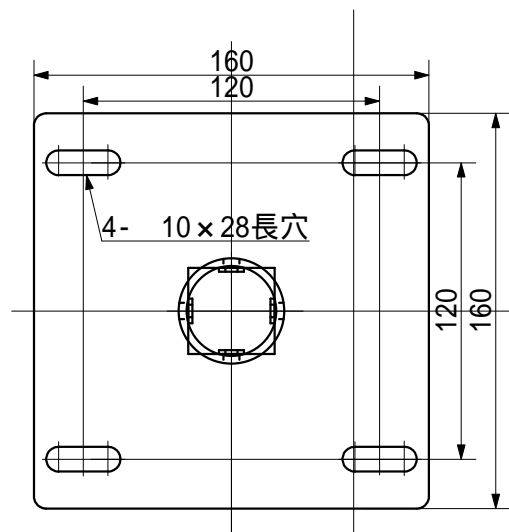
スラブ取付板
